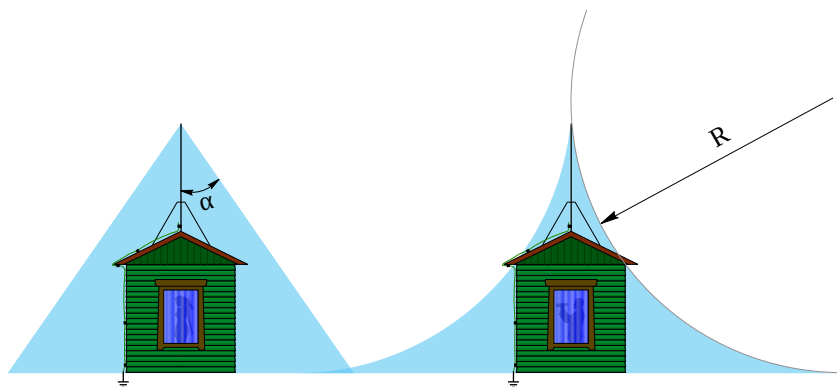
Рисунок 89 Область пространства, которую защищает молниеотвод. Удар в область отмеченную голубым цветом маловероятен, но не исключён. Слева использована методика защитного угла \alpha , величина которого берётся из стандарта МЭК 62305 в зависимости от высоты и требуемого уровня защиты. Справа использована методика катящейся сферы, радиус которой так же берётся из стандарта и зависит от высоты и требуемого уровня защиты.
