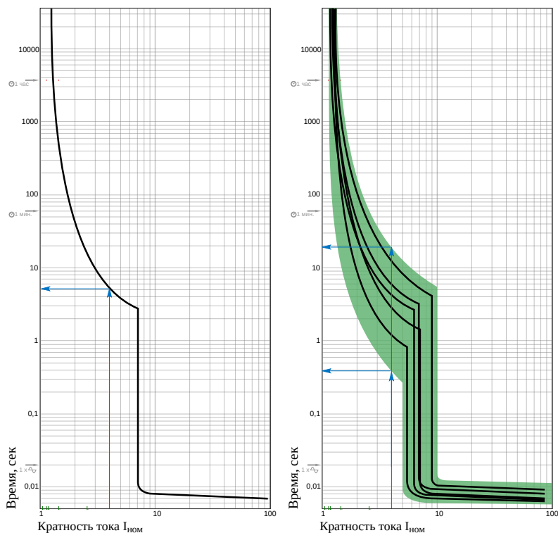
Рисунок 24 Слева изображён график времятоковой характеристики единичного экземпляра автоматического выключателя. Стрелками указано определение времени срабатывания при токе 4 \times I_{\text{ном}} , оно равно 5 секундам. Справа изображены времятоковые характеристики нескольких экземпляров автоматических выключателей и поле допуска, в которое укладывается любой взятый из партии автоматический выключатель. По графику видно, что при токе 4 \times I_{\text{ном}} время срабатывания автоматического выключателя будет от 0,4 до 20 сек.
