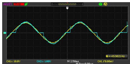
Рисунок 50 Форма тока с последовательным дуговым пробоем
